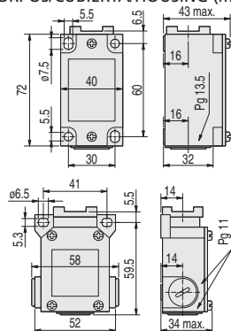
Fig. 1- CORPOS/CUBIERTA/HOUSING (mm)
