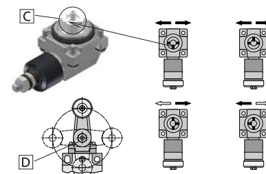
Fig. 6 - CABEÇOTE - OPÇÕES DE FUNCIONAMENTO/CABEZA - OPCIONES DE ACCIONAMIENTO/HEAD - OPERATION OPTIONS
