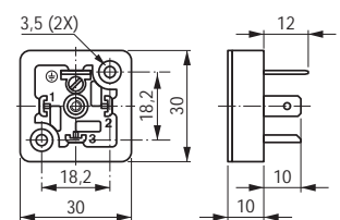
Base de Sobrepor tipo F (para conector quadrado)
