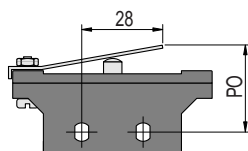
MFE - Alavanca Flexível
