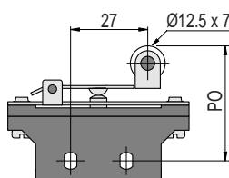
MFJ - Alavanca com Rolete
