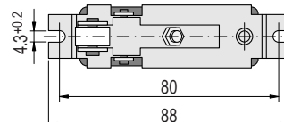
MFP - Alavanca c/ Rolete e Acionamento Invertido
