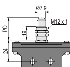
MFC - Atuador de Botão
