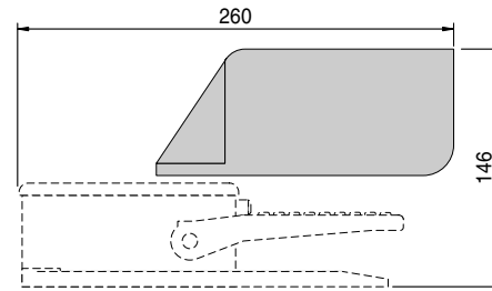
Protección SDB
