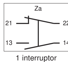
Esquema Eléctrico
